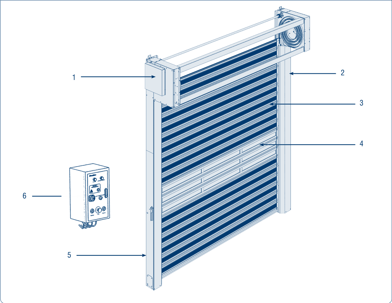
Рис. 1. Общий вид ворот
