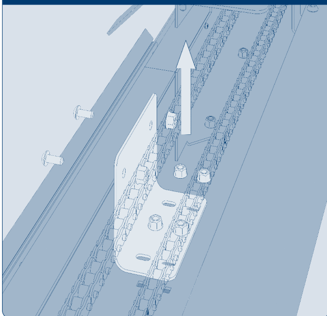
Рис. 14.1. Вид А
