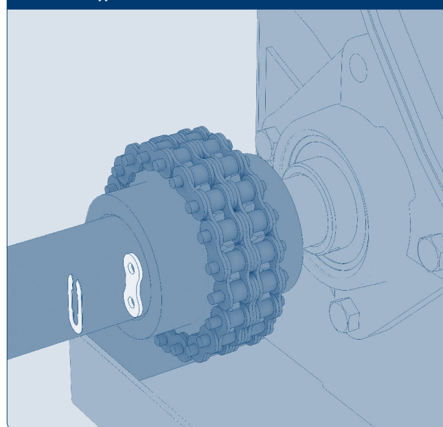
Рис. 5.2. Вид Б
