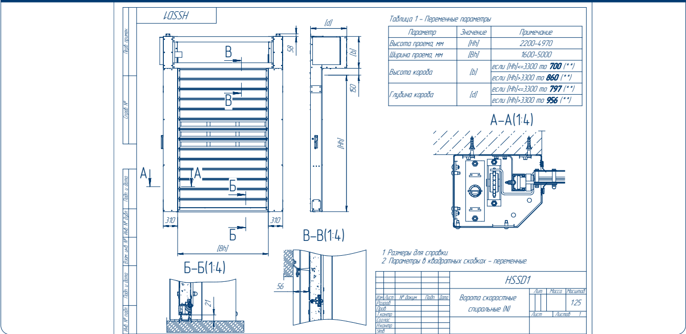
Рис. 2. Установочный чертеж
