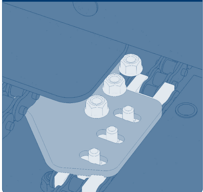
Рис. 12.1. Вид А
