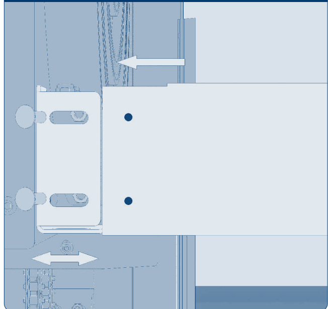
Рис. 6.2. Вид Б
