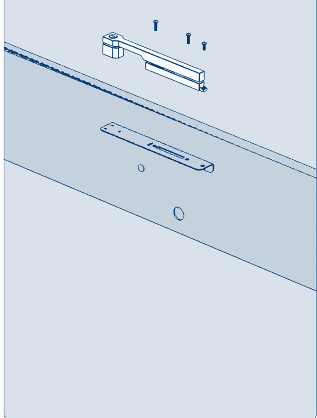
Рис. 3.1. Вид А
